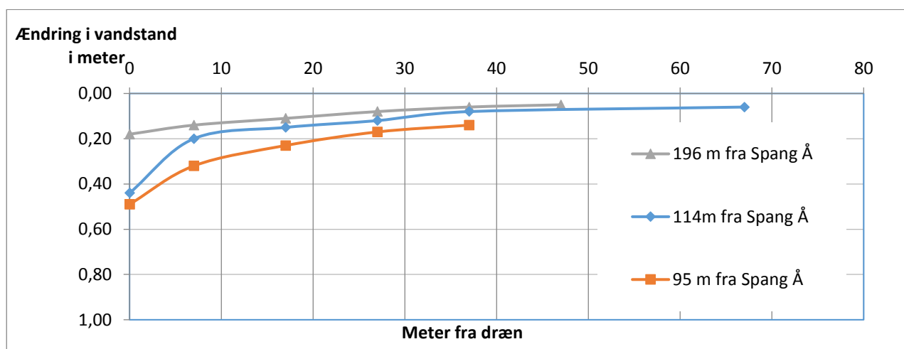
Figur 15. Vasby mose scenarie 2. Påvirkning af grundvandsspejl ved dræning med nedgravet drænrør i 0,50m dybde eller med åben grøft. Scenarie kørsler hvor trykniveau er påvirket med afstanden fra dræn.
