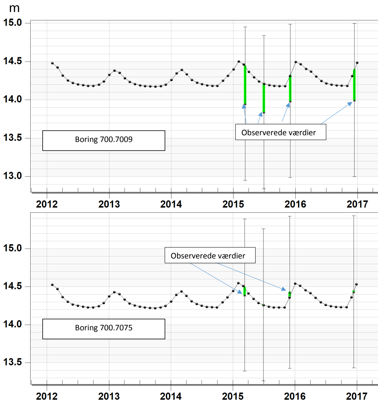
Figur 10 Figuren viser Riggilde modellens evne til at simulere de årlige variationer i trykniveau for perioden 2011-2016. Trekanten angiver observationer af vandstand i de to borer 700.7009 og 700.7075 i moserne. Boring 700.7009 (= VM3-1 i Vasby Mose der har filter i 1 meters dybde) og boring 700.7075 (= VM18-1 i Vasby Mose, der også har filter i 1 meters dybde). Kurverne med prikker viser de simulerede vandstandsvariationer i de to borer. De grønne stolper viser difference mellem observeret og simuleret vandstand.
