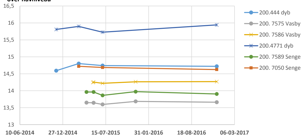
Figur 5. Afbildning af den tidslige variation i trykniveau for kalk- og sand-magasiner (dyb) og korte boringer filtersat i moseaflejringerne i hhv. Vasby og Sengeløse Moser.
