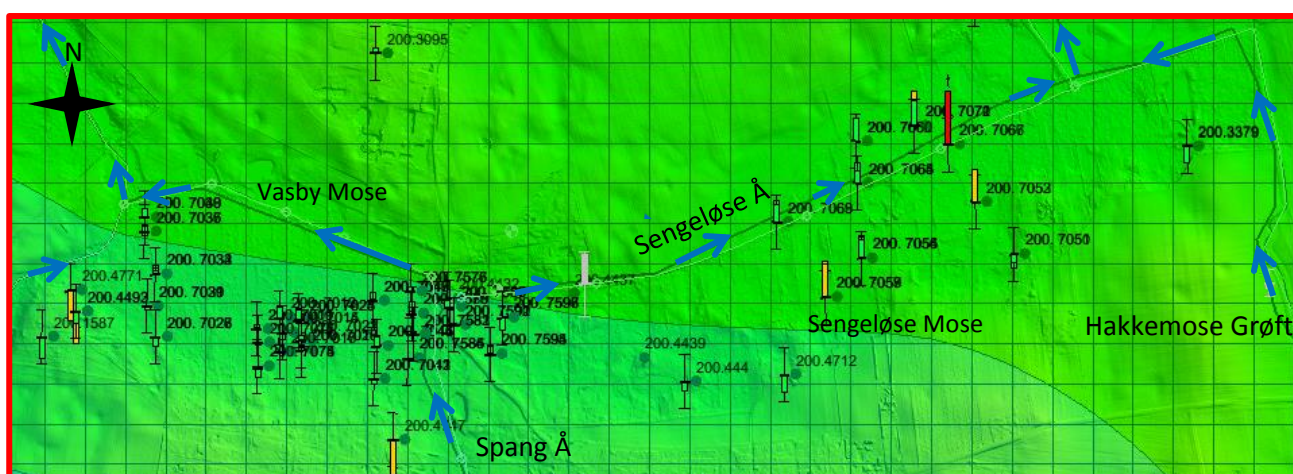
Figur 9 Kalibreret model og fejl på trykniveau (head) observationer. Størrelsen af søjlerne repræsenterer fejlen mellem simuleret og observeret trykniveau i de givne borer. Differensen imellem simuleret og observeret trykniveau er inddelt i tre farve kategorier: differens på 0-75 cm (grøn), differens på 75-150 cm (gul) og differens > 150 cm (rød). Potentialelinjer er optegnet på baggrund af Store Pejledag 2016 målingerne. Nederst er vist et zoom af området ved selve moserne.
