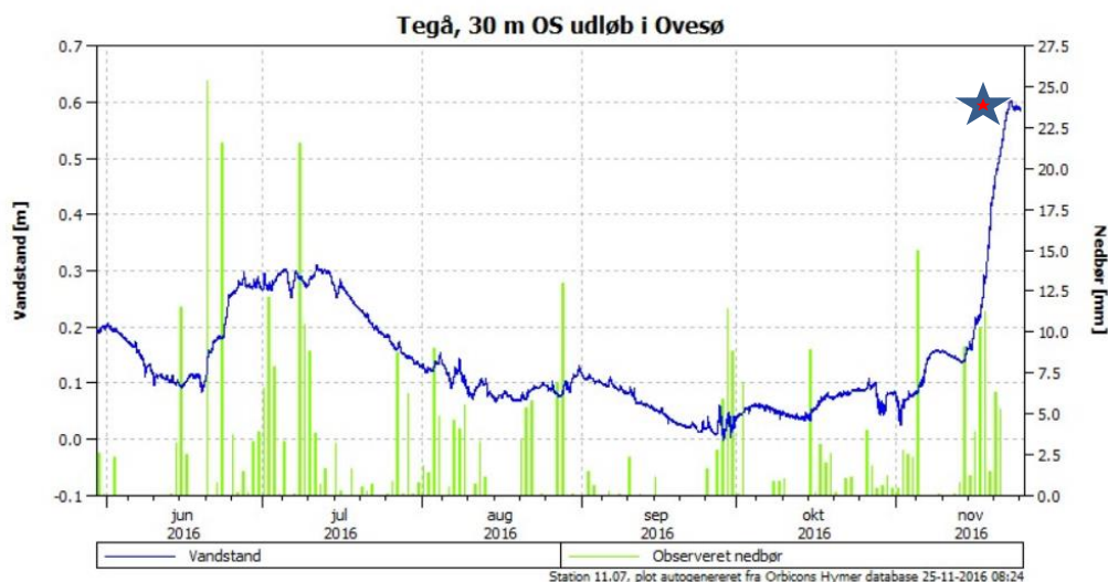
Figur 4-31. Vandstand og nedbør. Udløb af Tegå i Ove Sø. Bemærk skala på vandstand forkeret. Man kan sammenligne kurven fra juni til august med Figur 4-32. Data Orbicon.
