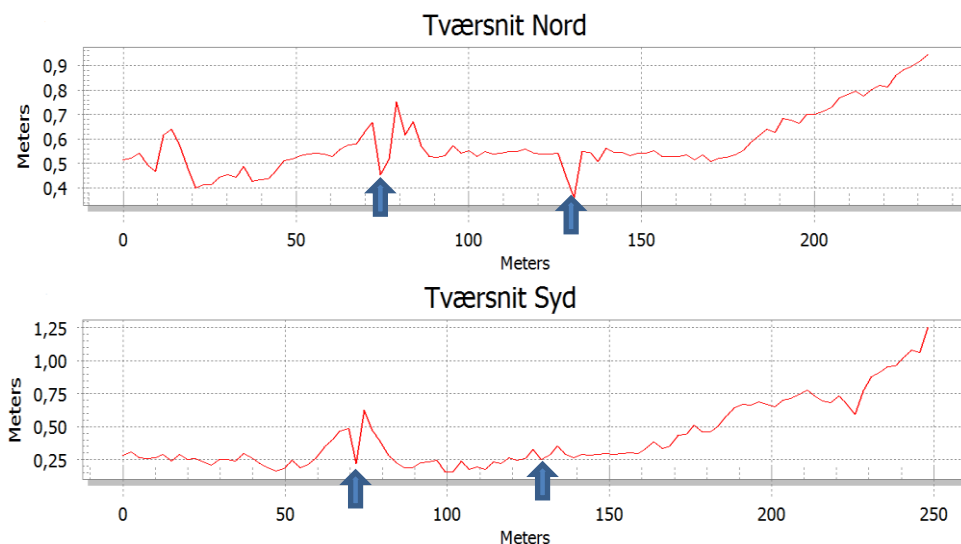
Figur 6-13. Øverst: tværsnit V-Ø over Å og gl forløb, ca. 130m. nedstrøms hovedvejen. Nederst: tværsnit V-Ø over Å og gl forløb ca. 225m. nedstrøms hovedvejen. Pile til venstre er Mølleåen, til højre det gamle forløb.
