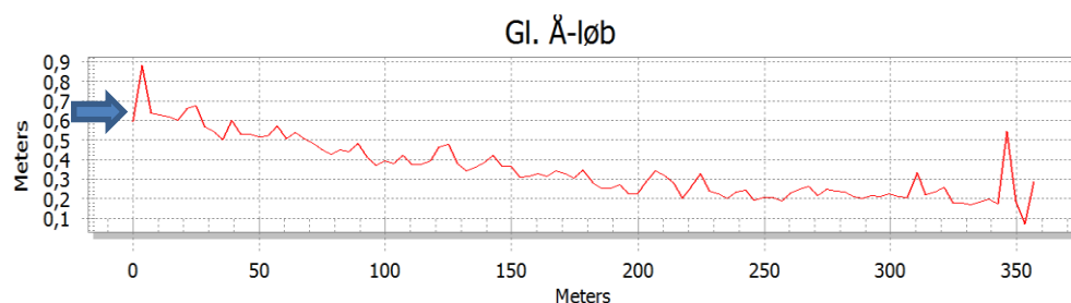
Figur 6-14. Terrænforhold gennem det gamle åløb, fra nord mod syd, målt i DHM
