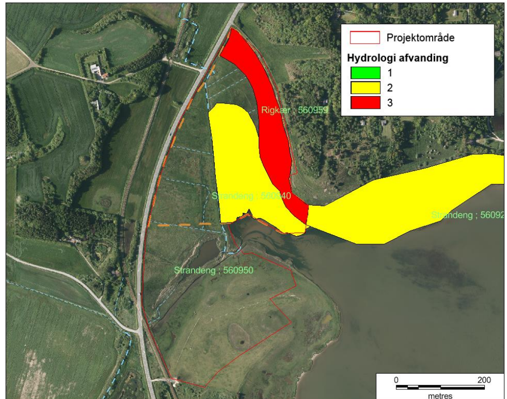
Figur 5-5. Hydrologi 2011. 1: ingen afvanding, 2: nogen afvanding, 3: stærkt afvandet
