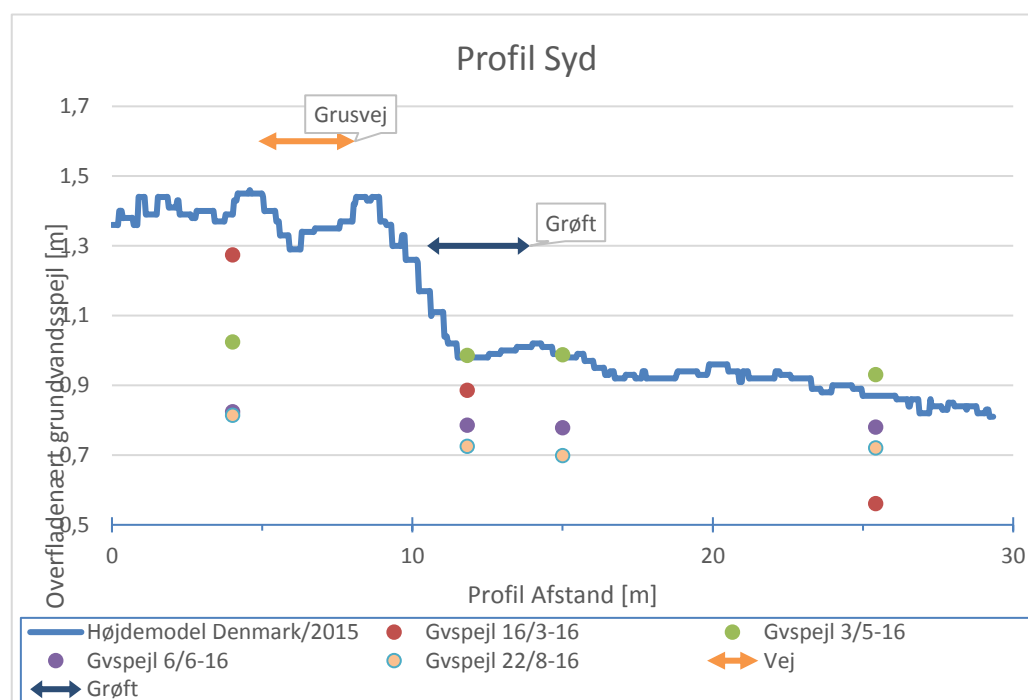
Figur 6-11. Terrænprofil og observerede vandspejl i etablerede borer på profil Syd.
