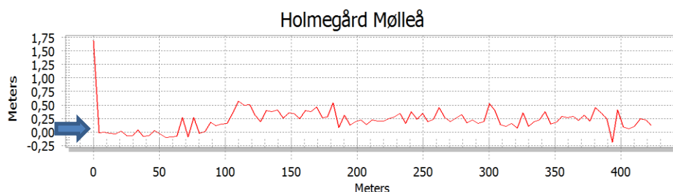
Figur 6-15. Vandspejl for Holmegårde Mølleå, fra hovedvejen i nord til udløb i syd, målt i DHM
