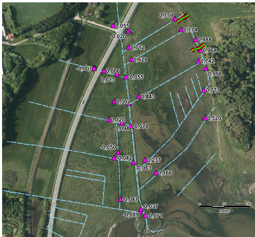
Figur 5-1. Supplerende vandstandsmålinger maj 2016. Blå streg: grøfter, lilla trekant: bundkoter i grøfter, røde ruder og grøn streg: grundvandspejlinger.
