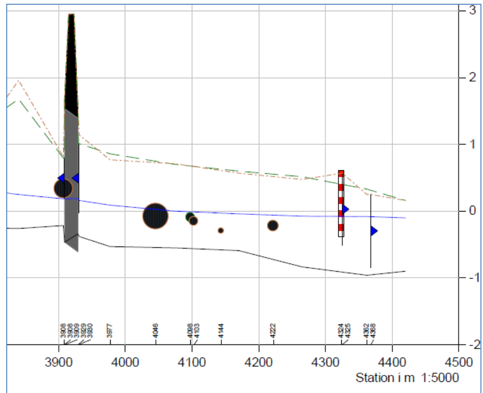
Figur 5-21. VASP-plot. Det ses, at vandløbsbundens kote (sort) ved hovedvejen (mørk kegle til venstre) er ca. -0,4\text{m.} , og falder ned til udløbet til ca. -1\text{m.} Vandspejl (blå) ligger i ca. 0,2\text{m.} ved hovedvejen og lidt under 0\text{m.} ved udløbet. Koter i DVR90. Grøn og orange stiplede linje er kote for hhv. højre og venstre brink.
