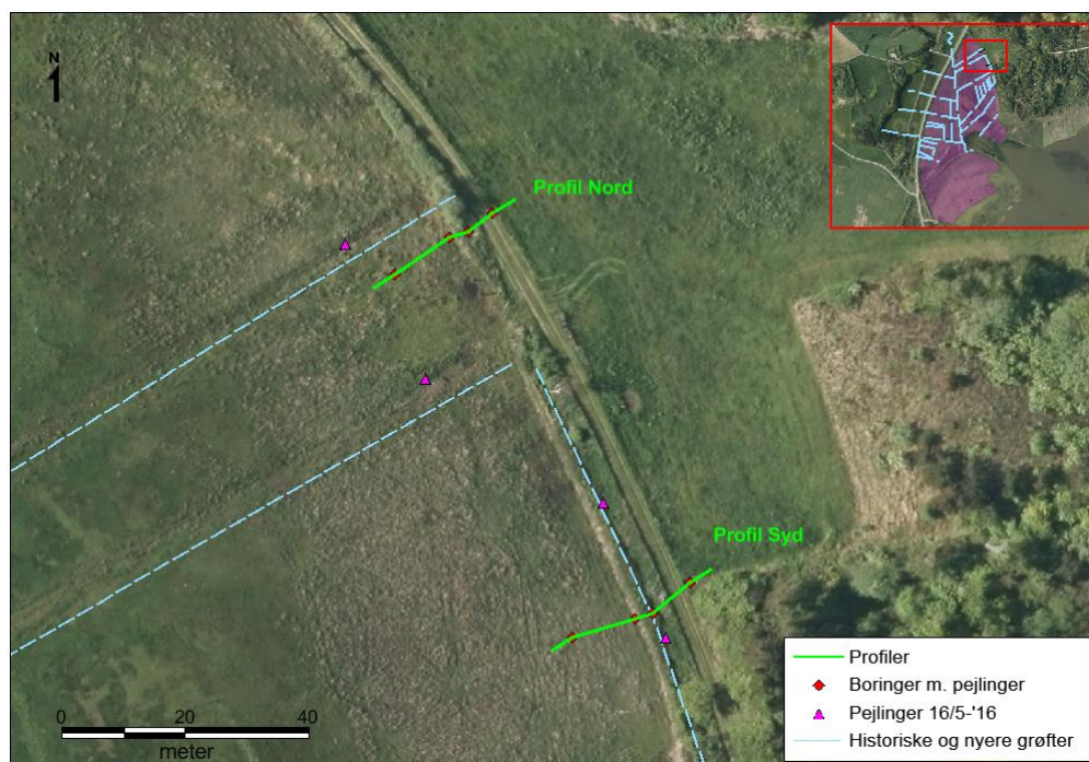
Figur 6-9. Boringer hvor det overfladenære grundvandsspejl er målt i løbet af foråret og sommeren 2016. Desuden er vist supplerende målinger af grundvandsspejlet fra maj 2016.
