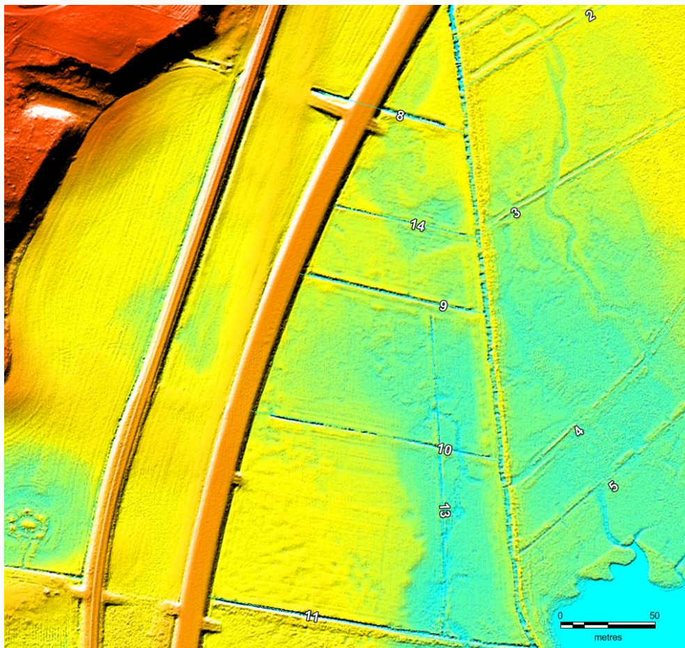
Figur 7-3. Højdemodel DHM. Grøfterne er nummereret.
