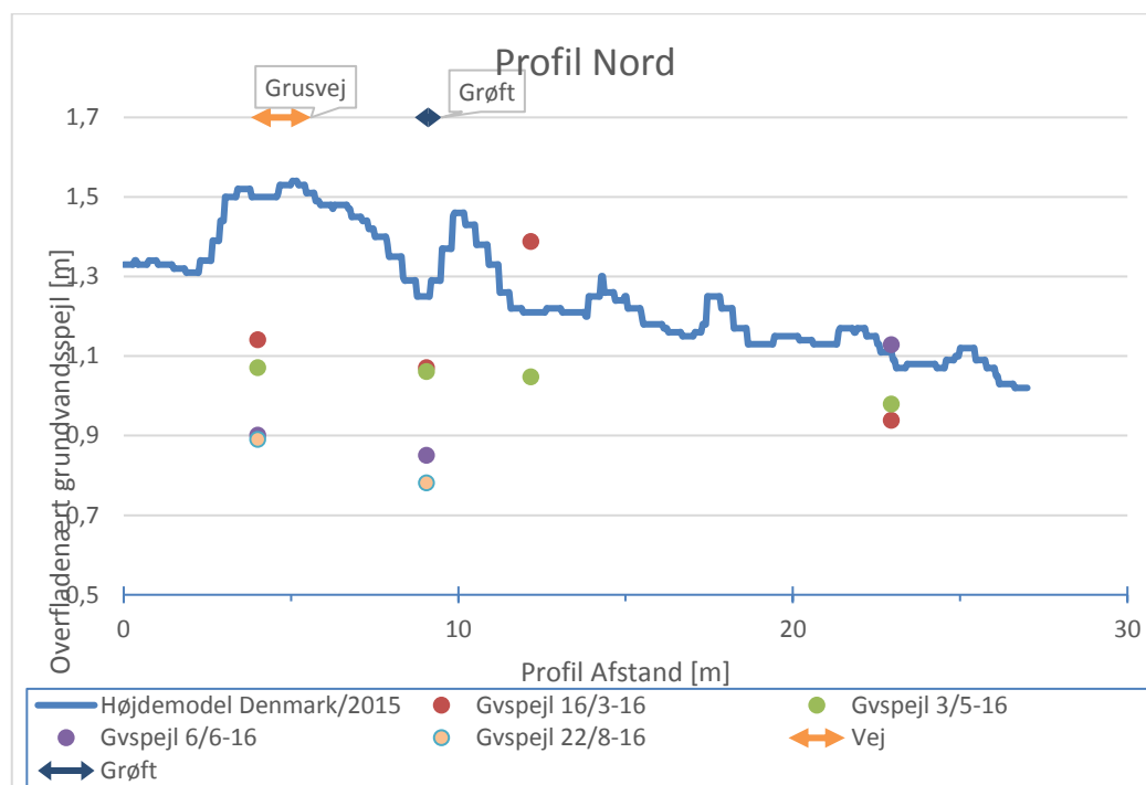
Figur 6-10. Terrænprofil og observerede vandspejl i etablerede borer på profil Nord.
