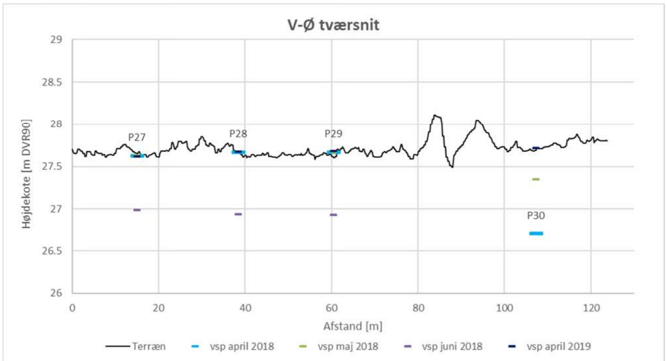
Figur 4-21 Pejleprofil i delområde 7. Den nordlige del af Centralgrøften ses til højre (for P30).
